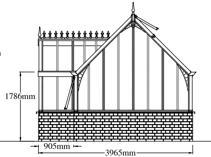
RIGHT ELEVATION
