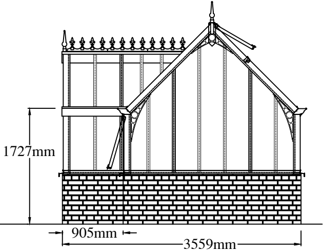
RIGHT ELEVATION
