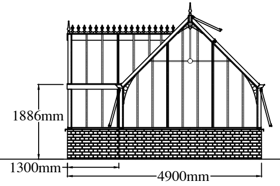
RIGHT ELEVATION
